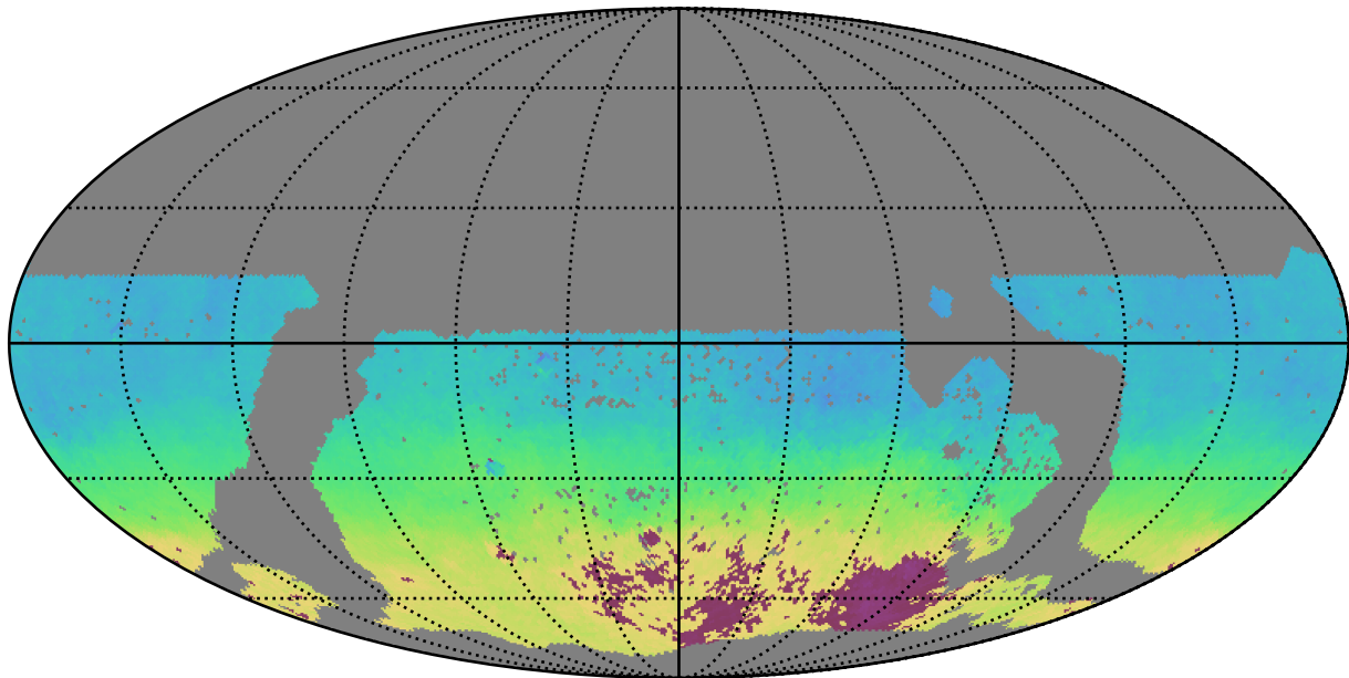
mw_roll_all_v3.3_10yrs WFD y band: AngleMean rotSkyPos
