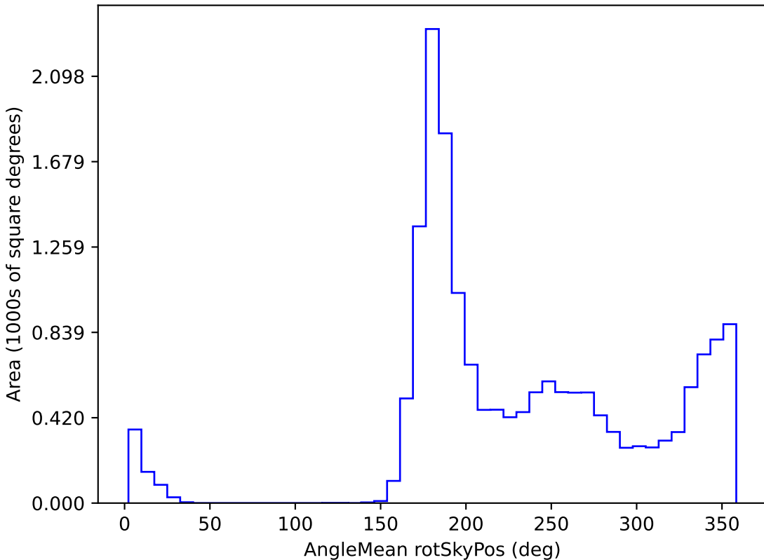
mw_roll_all_v3.3_10yrs WFD y band: AngleMean rotSkyPos
