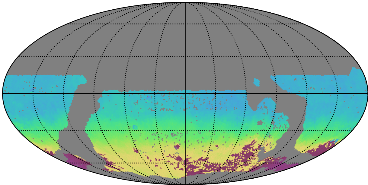
mw_roll_all_v3.3_10yrs WFD i band: AngleMean rotSkyPos
