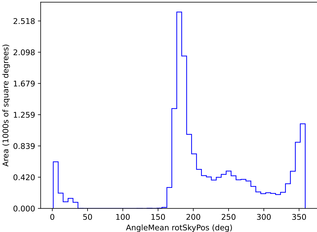
mw_roll_all_v3.3_10yrs WFD i band: AngleMean rotSkyPos
