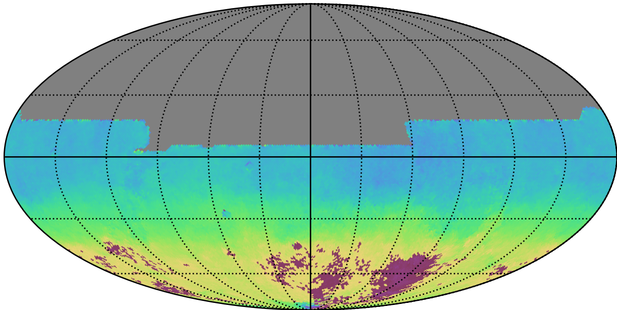
mw_roll_all_v3.3_10yrs All sky y band: AngleMean rotSkyPos
