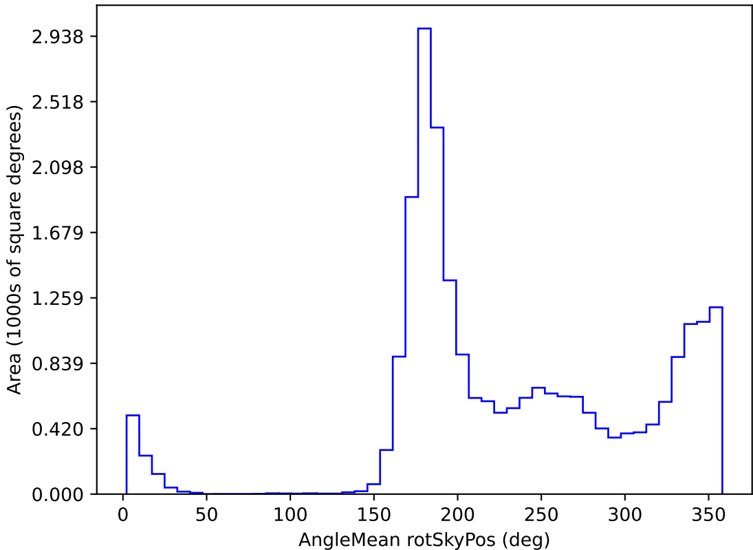
mw_roll_all_v3.3_10yrs All sky y band: AngleMean rotSkyPos
