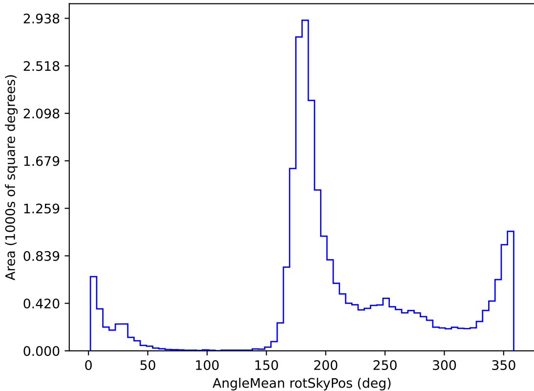
mw_roll_all_v3.3_10yrs All sky i band: AngleMean rotSkyPos
