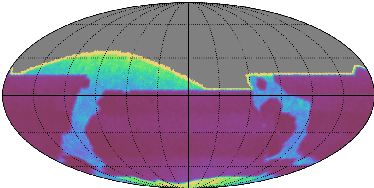
mw_roll_all_v3.3_10yrs : properMotion
