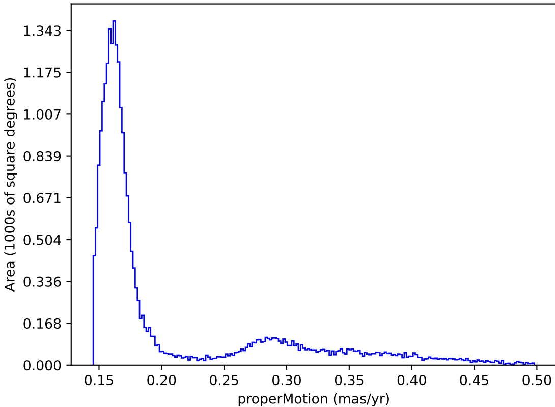
mw_roll_all_v3.3_10yrs : properMotion
