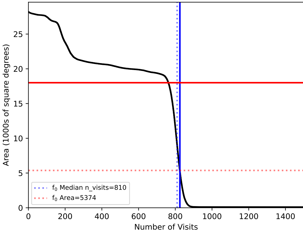
mw_roll_all_v3.3_10yrs : f0
