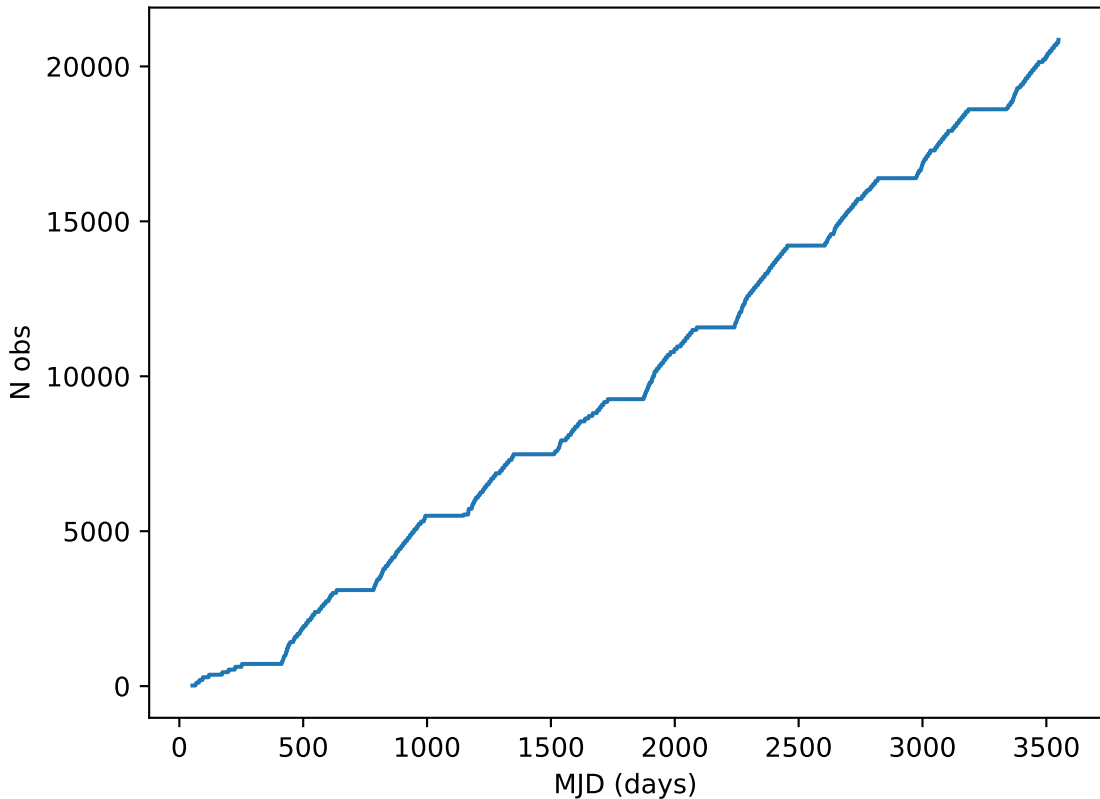
mw_roll_all_v3.3_10yrs note like DD:ELAISS1%: Cumulative
