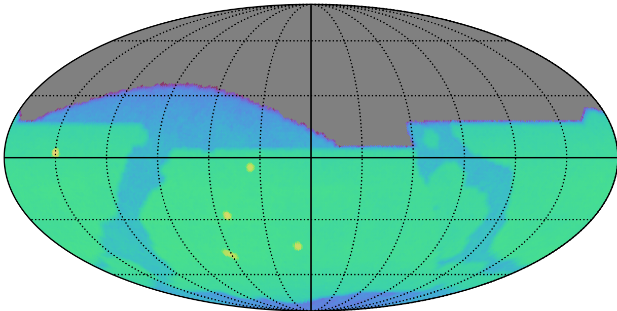
mw_roll_all_v3.3_10yrs z: CoaddM5
