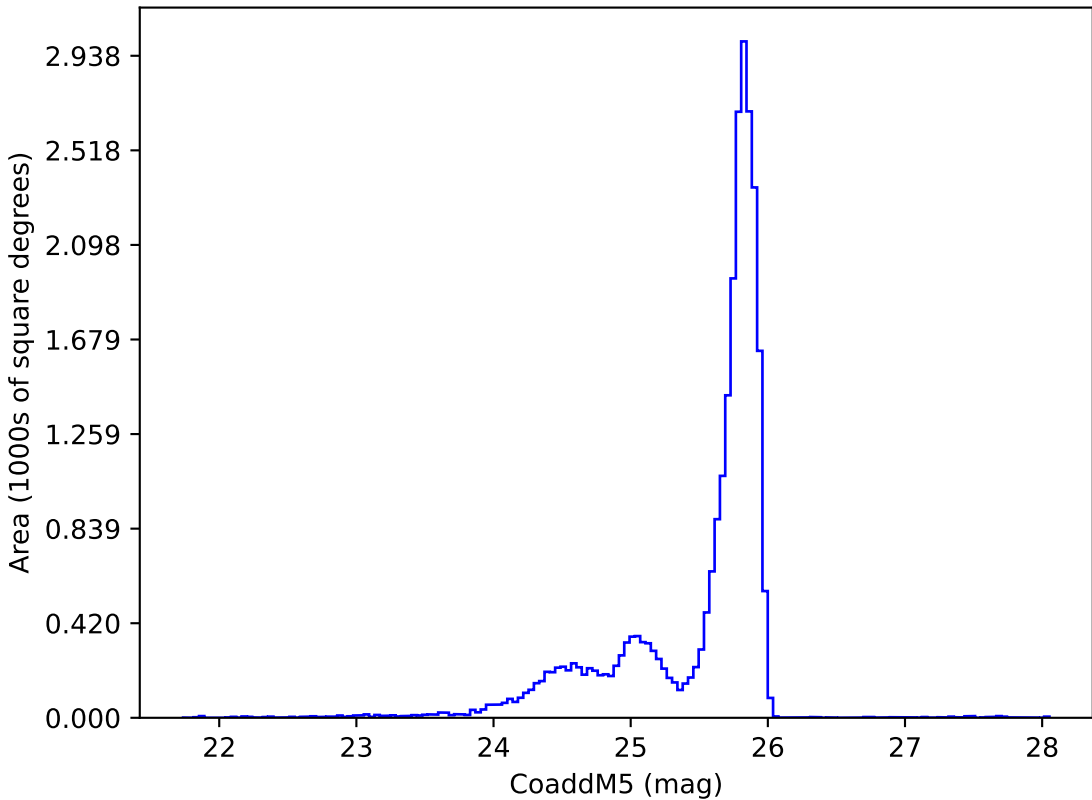
mw_roll_all_v3.3_10yrs z: CoaddM5
