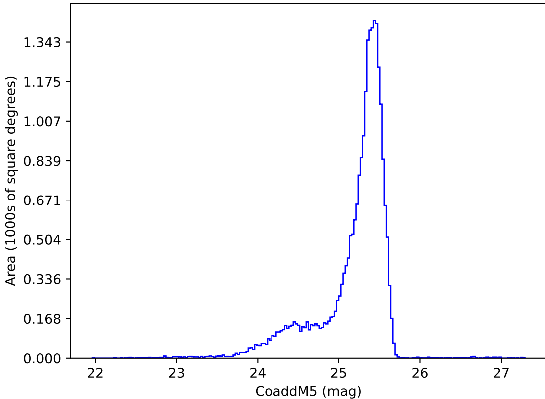
mw_roll_all_v3.3_10yrs u: CoaddM5
