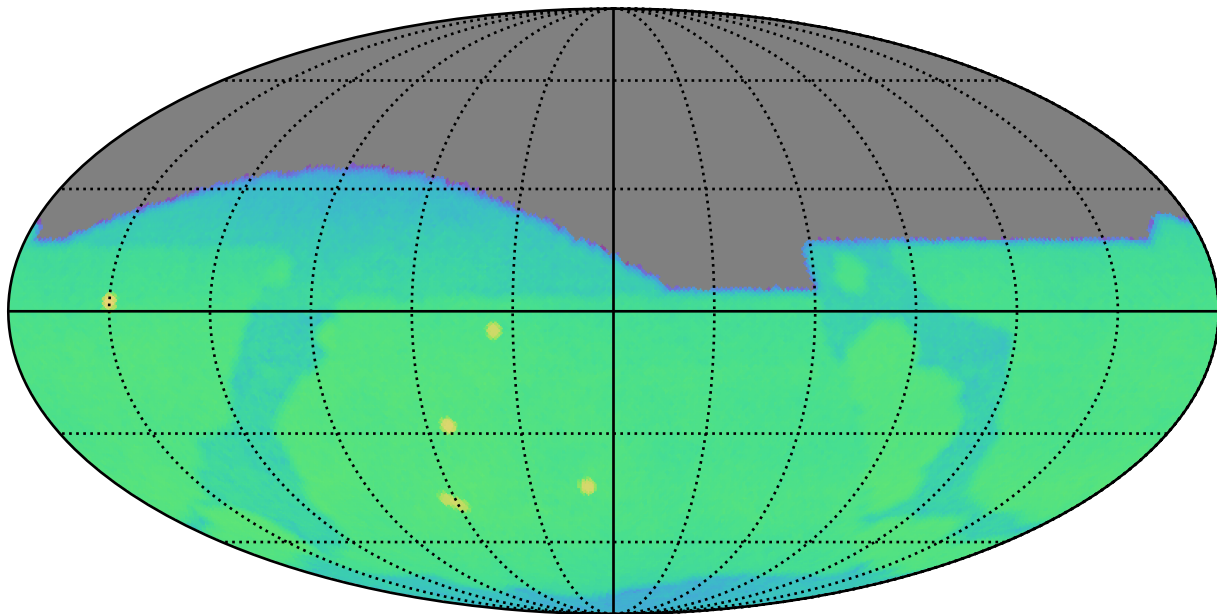
mw_roll_all_v3.3_10yrs g: CoaddM5
