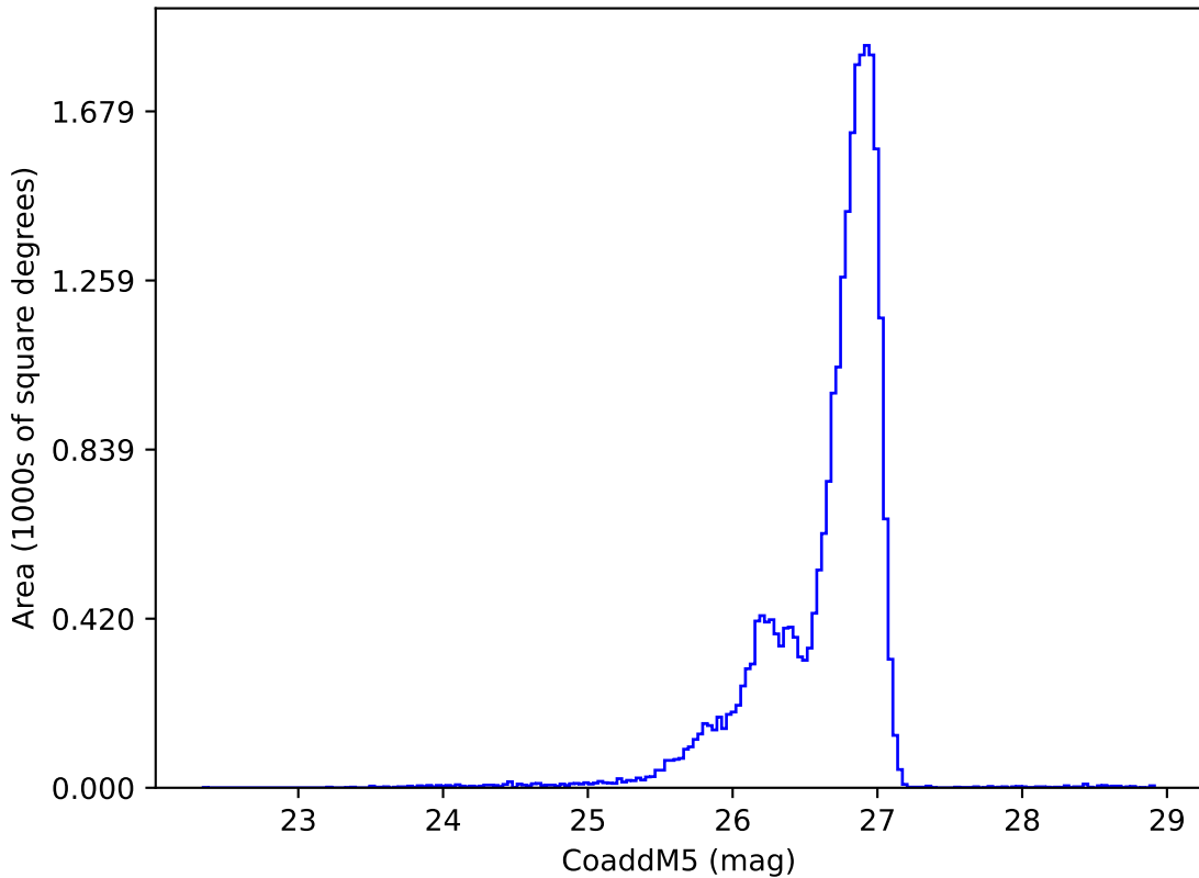
mw_roll_all_v3.3_10yrs g: CoaddM5
