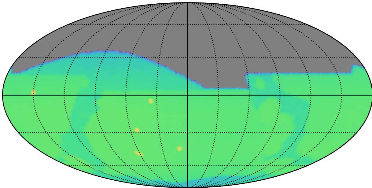
mw_roll_all_v3.3_10yrs : CoaddM5
