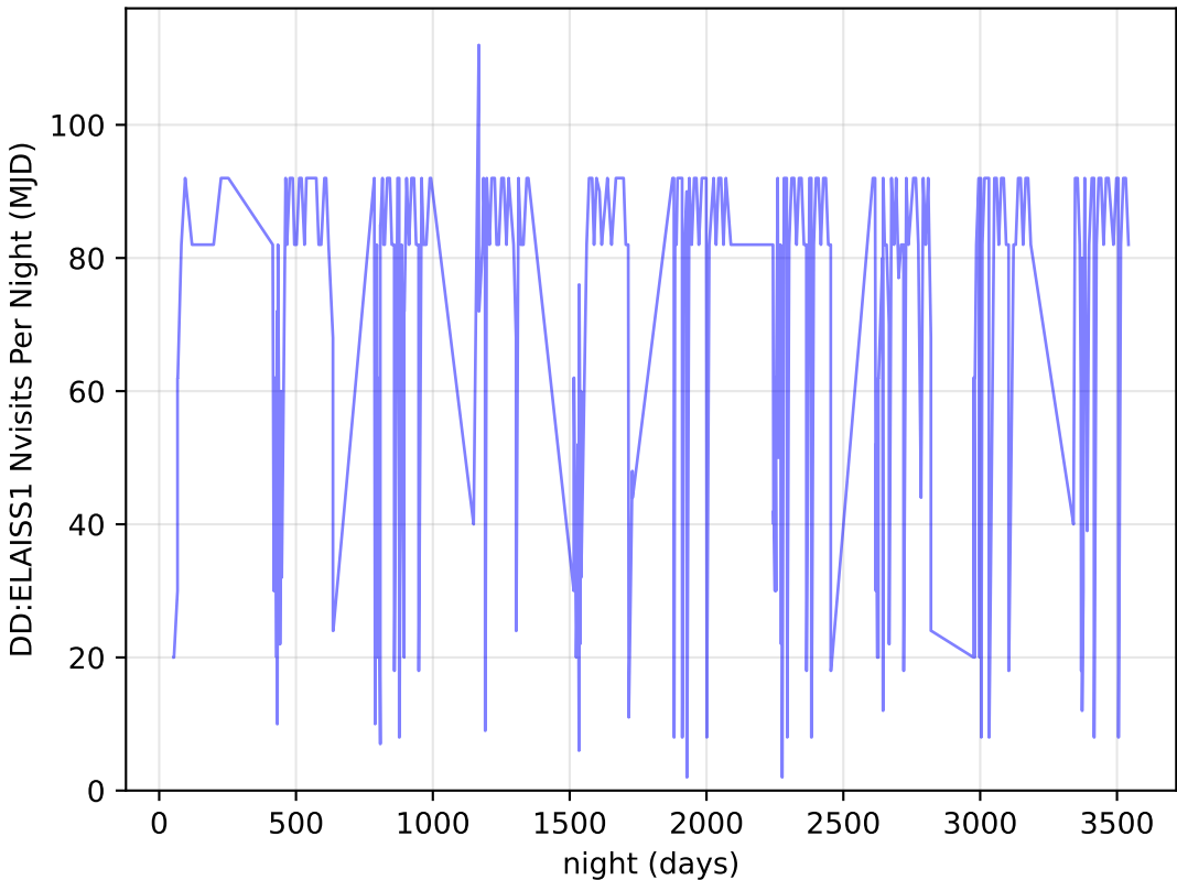
mw_roll_all_v3.3_10yrs all bands: DD:ELAISS1 Nvisits Per Night
