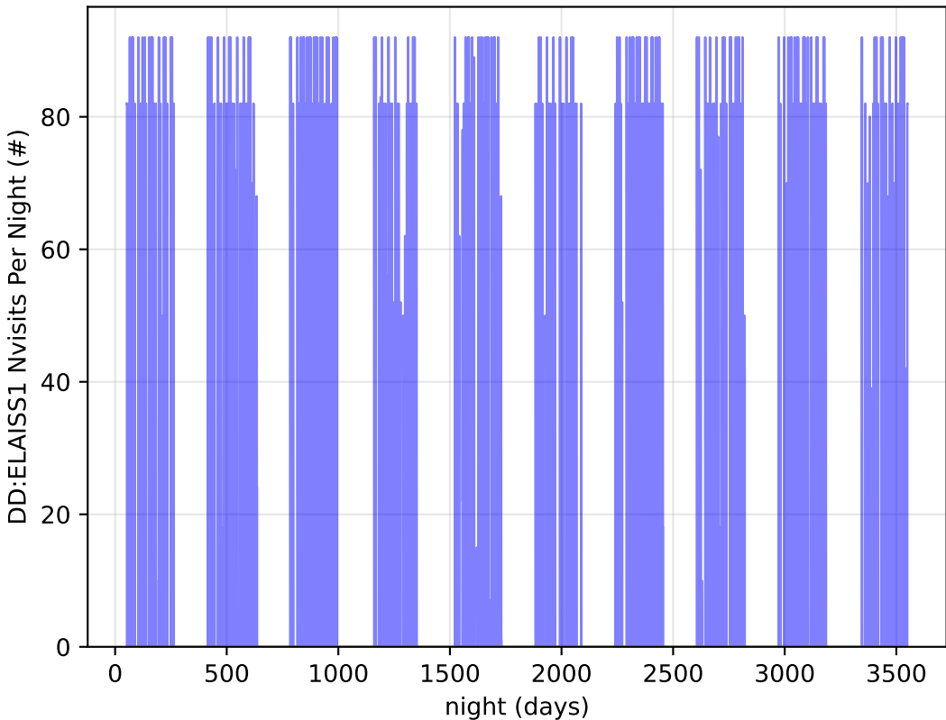
Imc_filter_balance_v3.4_10yrs all bands: DD:ELAISS1 Nvisits Per Night
