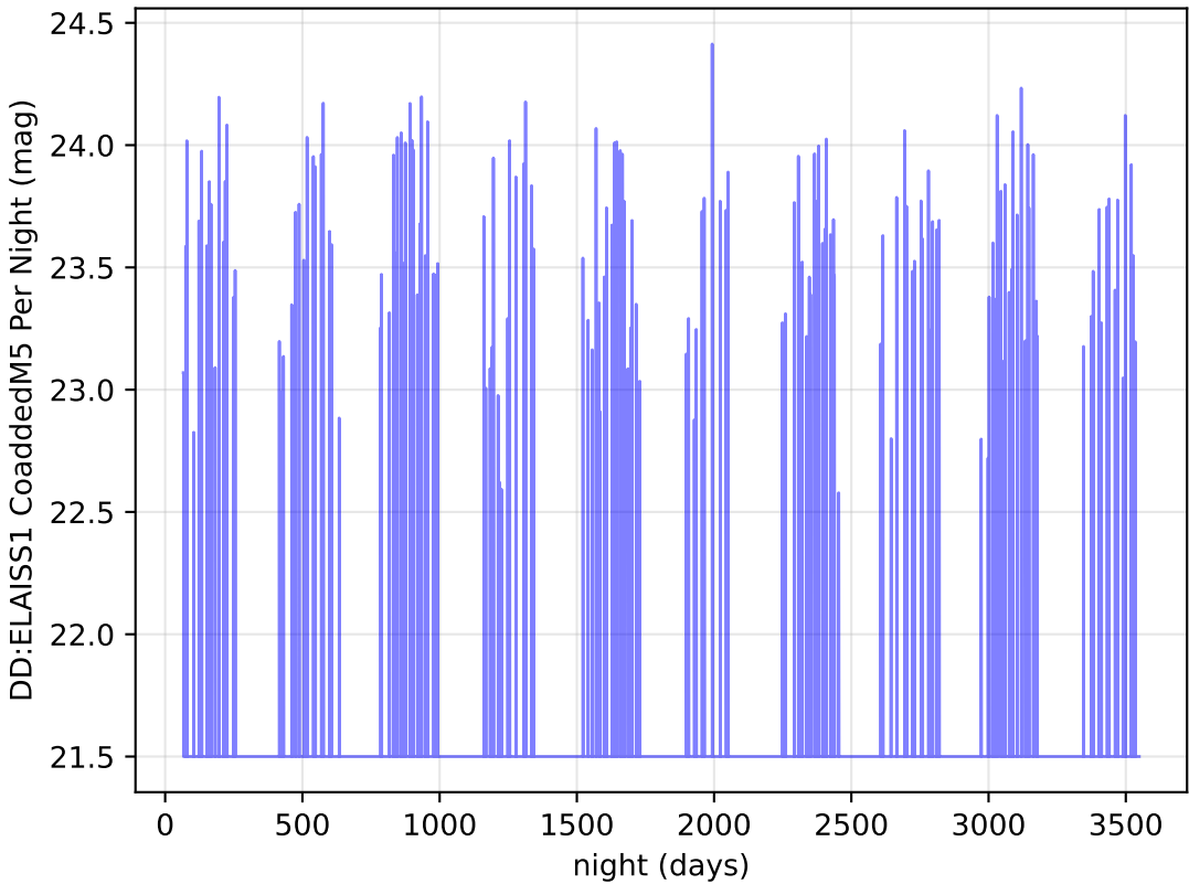
Imc_filter_balance_v3.4_10yrs y band: DD:ELAISS1 CoaddedM5 Per Night
