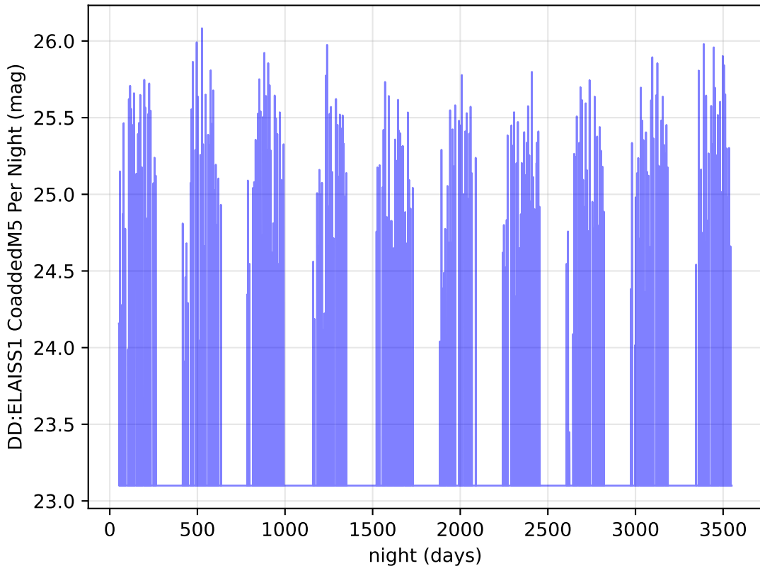
Imc_filter_balance_v3.4_10yrs i band: DD:ELAISS1 CoaddedM5 Per Night
