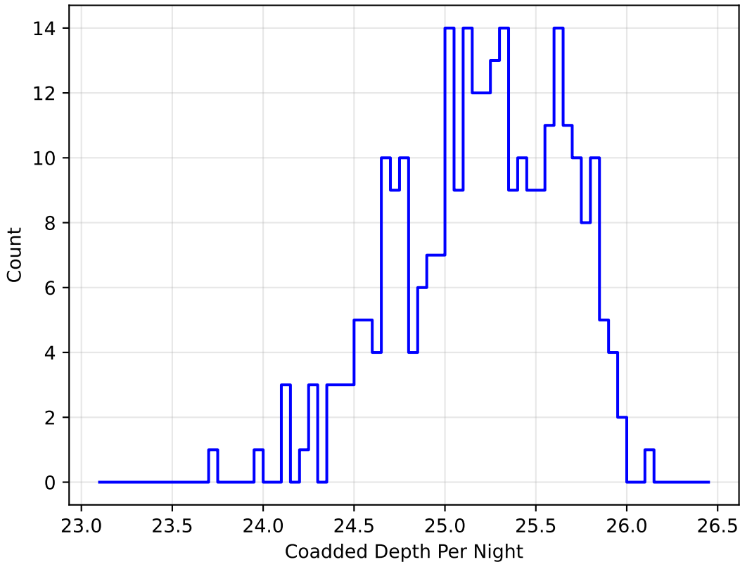
Imc_filter_balance_v3.4_10yrs i band: DD:EDFS CoaddM5PerNight
