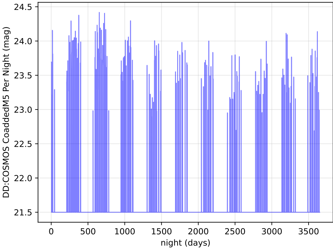
Imc_filter_balance_v3.4_10yrs y band: DD:COSMOS CoaddedM5 Per Night
