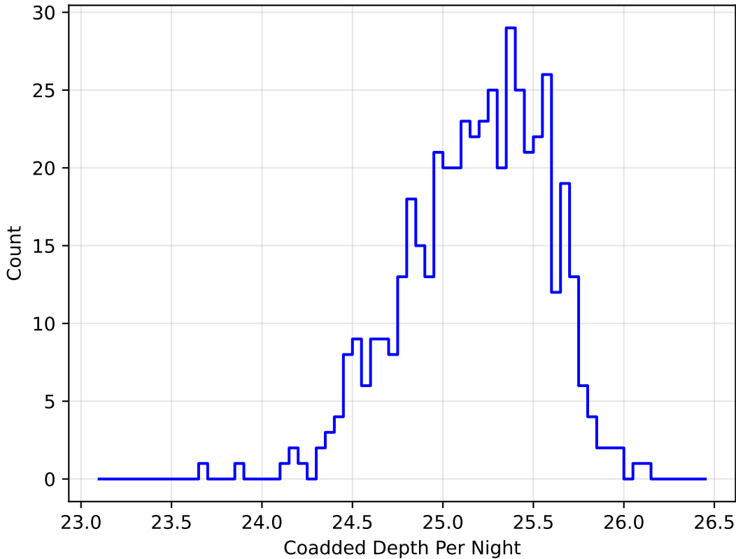
Imc_filter_balance_v3.4_10yrs i band: DD:COSMOS CoaddM5PerNight
