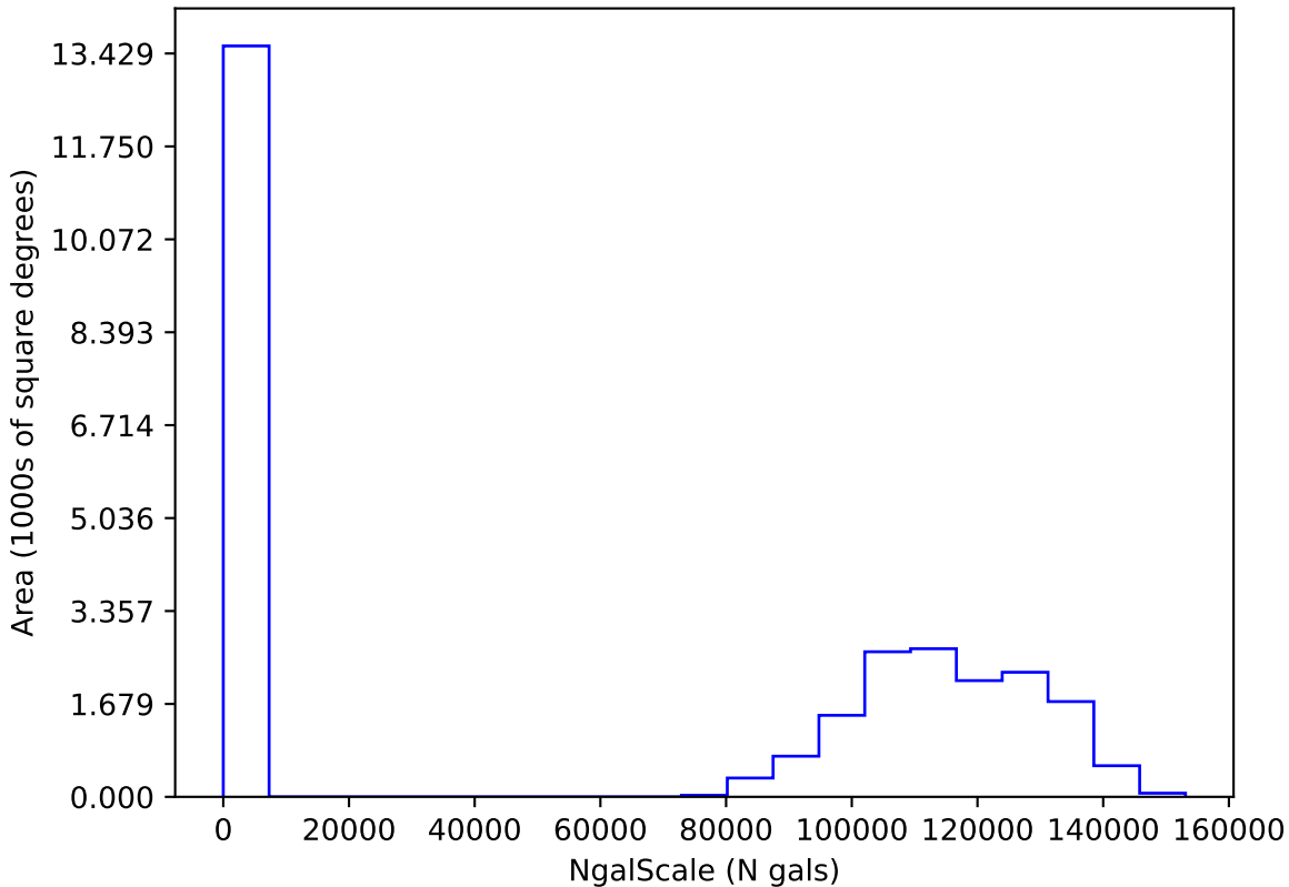
internal_u_expt45_nscale1.5v3.4_10yrs i: NgalScale
