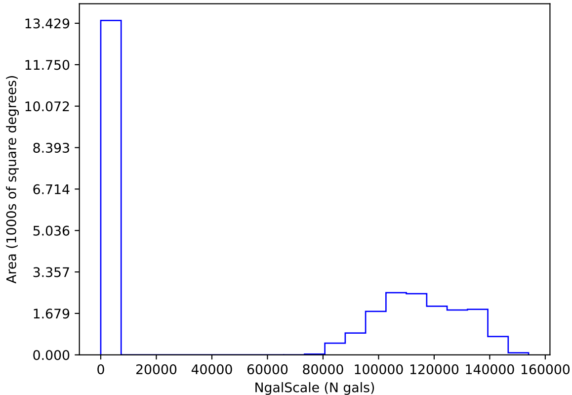
internal_u_expt45_nscale1.2v3.4_10yrs i: NgalScale
