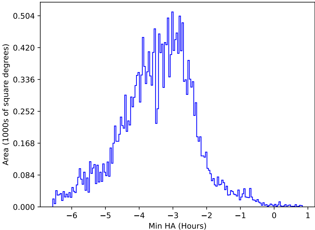
internal_u_expt45_nscale0.9v3.4_10yrs All sky y band: Min HA
