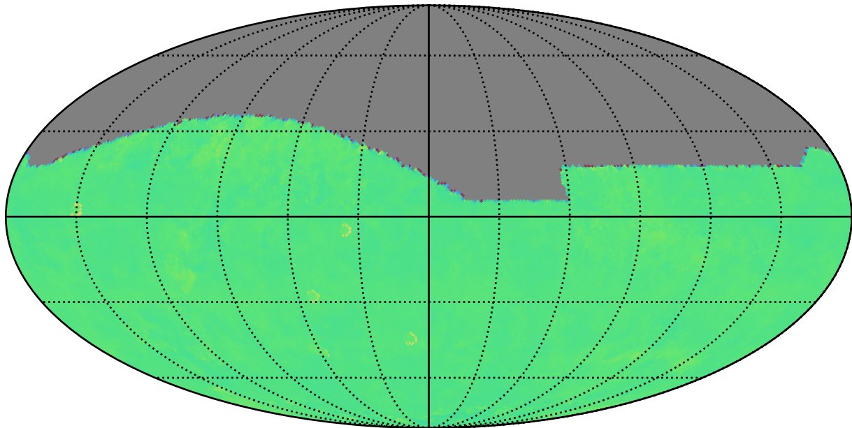
internal_u_expt38_nscale1.5v3.4_10yrs i: Kuiper rotTelPos
