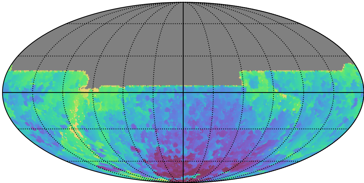
internal_u_expt38_nscale1.5v3.4_10yrs All sky y band: Min HA
