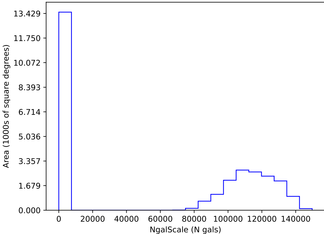
internal_u_expt38_nscale1.0v3.4_10yrs i: NgalScale
