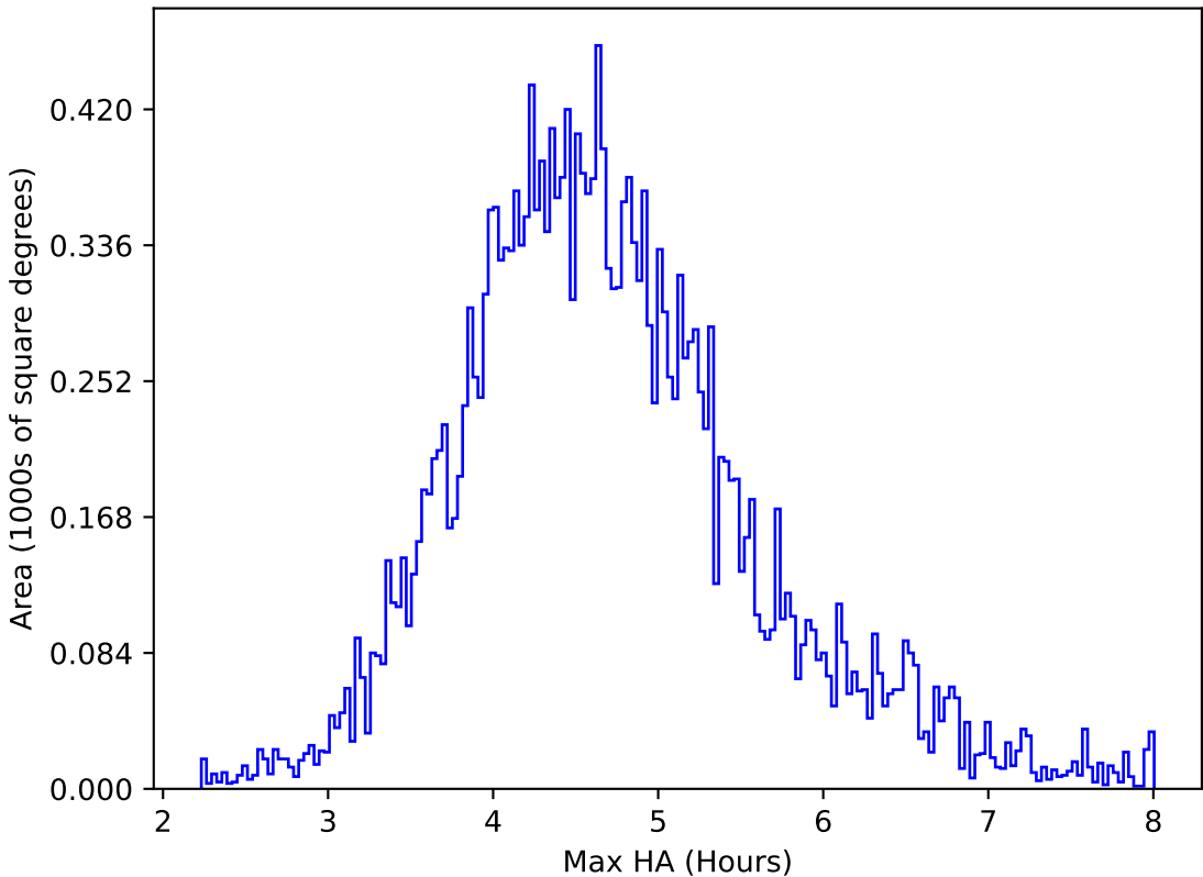
internal_u_expt38_nscale1.0v3.4_10yrs All sky y band: Max HA
