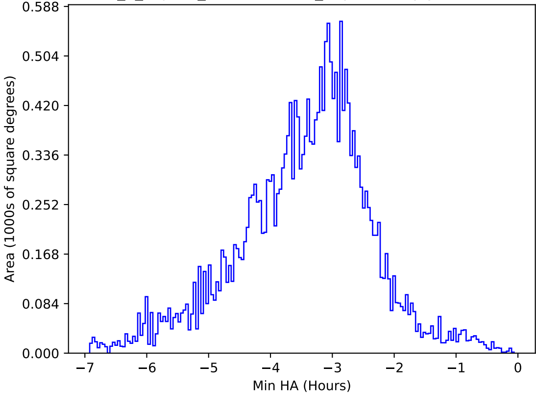
internal_u_expt38_nscale0.9v3.4_10yrs All sky y band: Min HA
