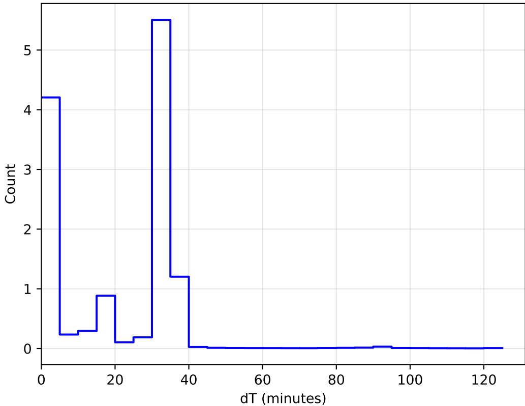
internal_u_expt38_nscale0.9v3.4_10yrs All sky: DeltaT Histogram 1e6
