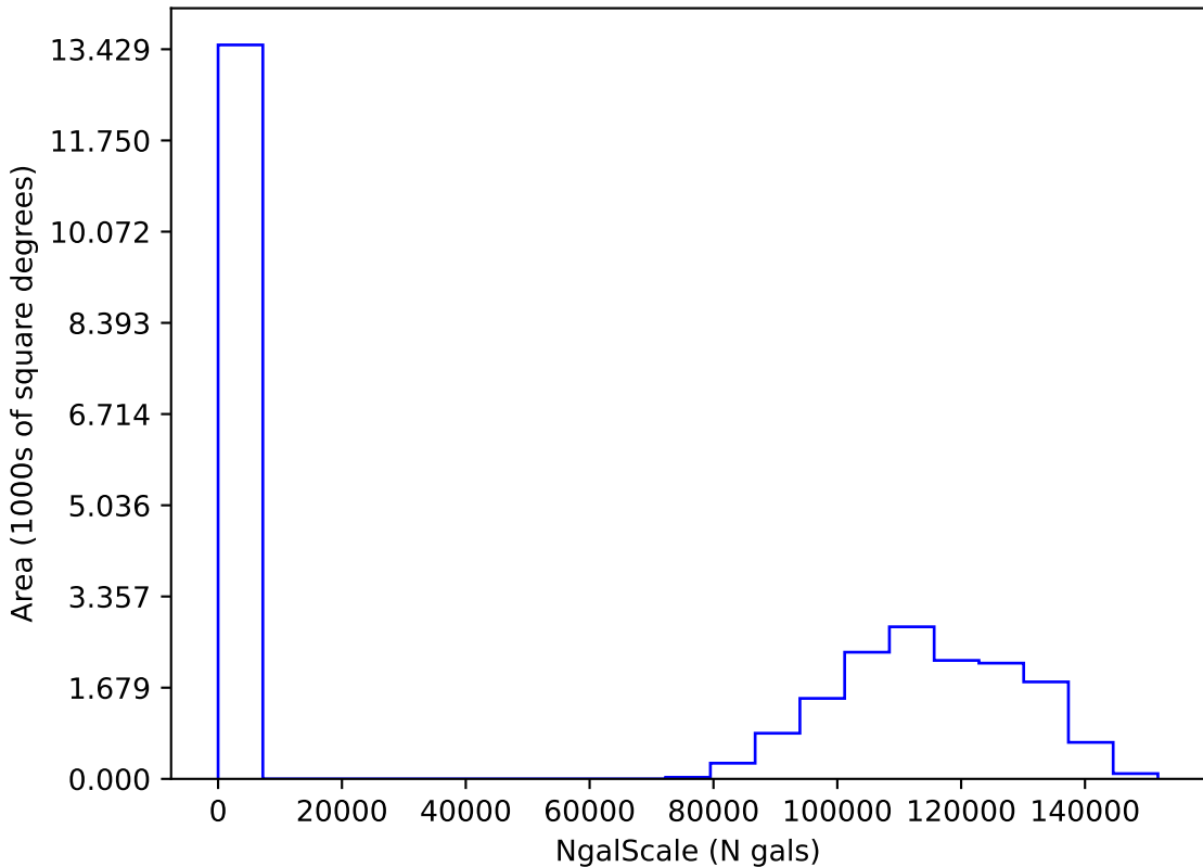
internal_u_expt30_nscale1.1v3.4_10yrs i: NgalScale
