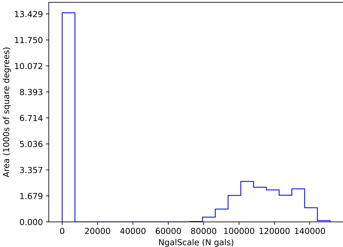
internal_u_expt30_nscale1.0v3.4_10yrs i: NgalScale
