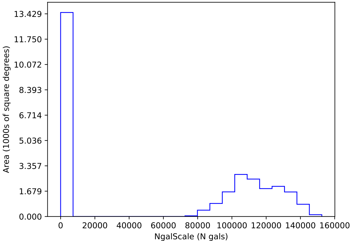
internal_u_expt30_nscale0.9v3.4_10yrs i: NgalScale
