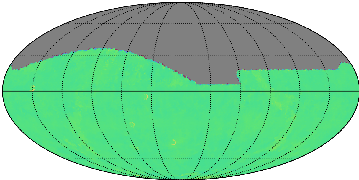
internal_u_expt30_nscale0.9v3.4_10yrs i: Kuiper rotTelPos
