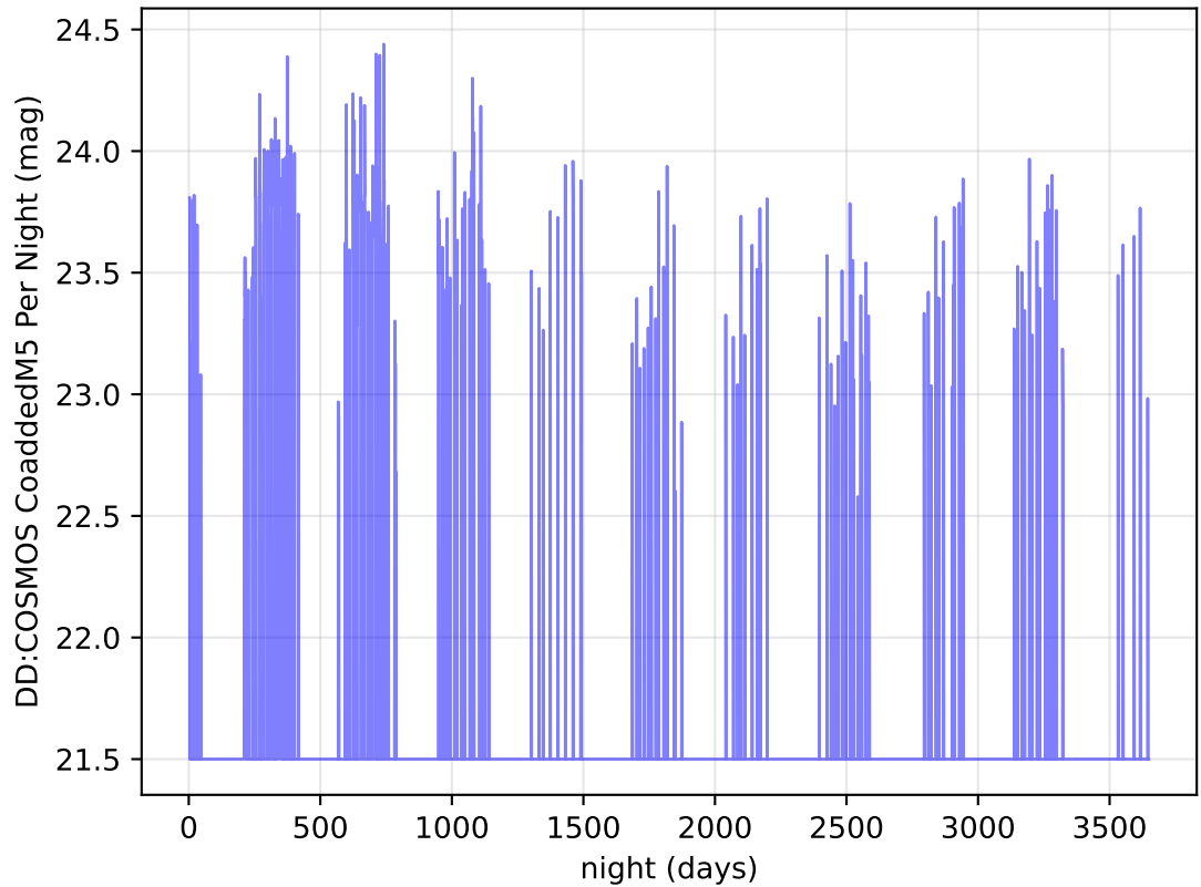
internal_u_expt30_nscale0.9v3.4_10yrs y band: DD:COSMOS CoaddedM5 Per Night
