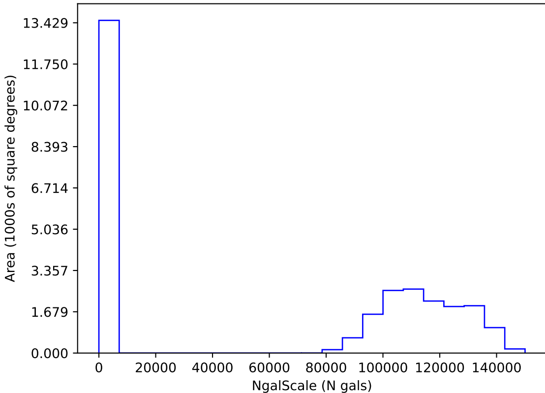
internal_u_expt27_nscale1.2v3.4_10yrs i: NgalScale
