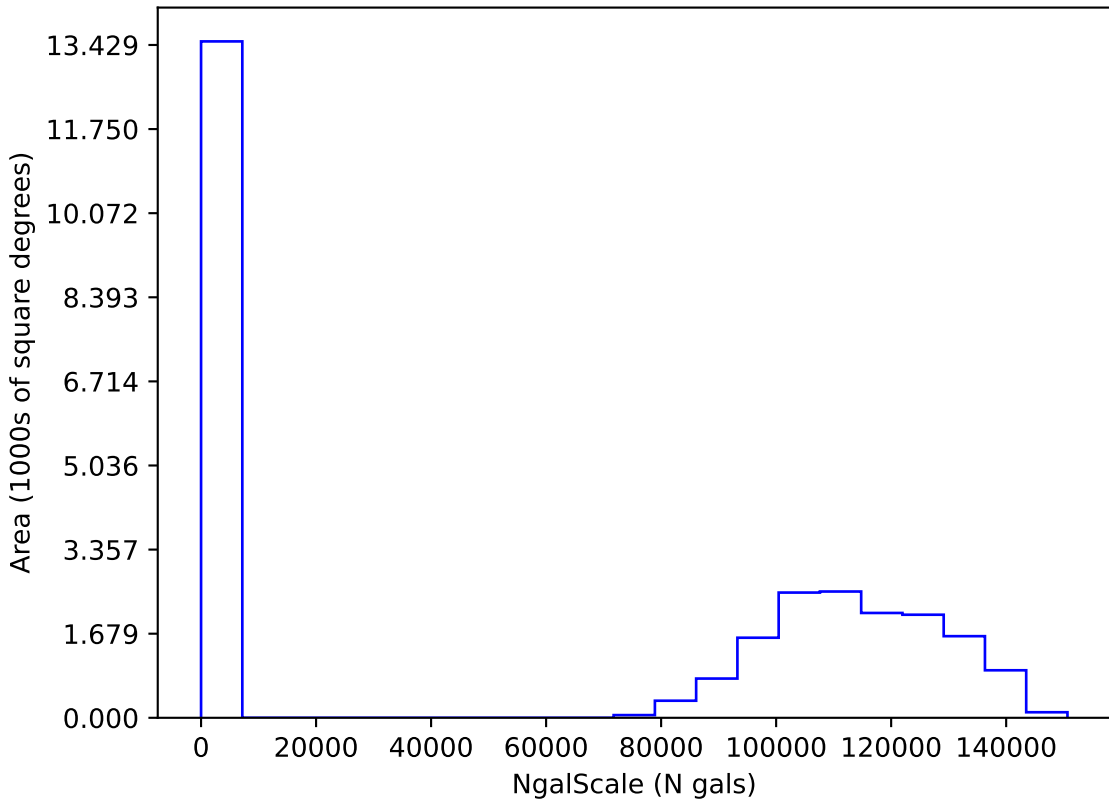
internal_u_expt27_nscale0.9v3.4_10yrs i: NgalScale
