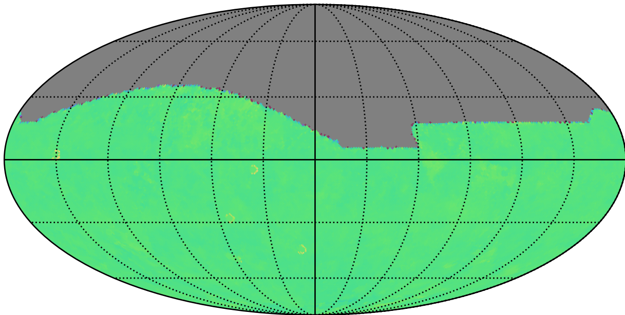
internal_u_expt27_nscale0.9v3.4_10yrs i: Kuiper rotTelPos
