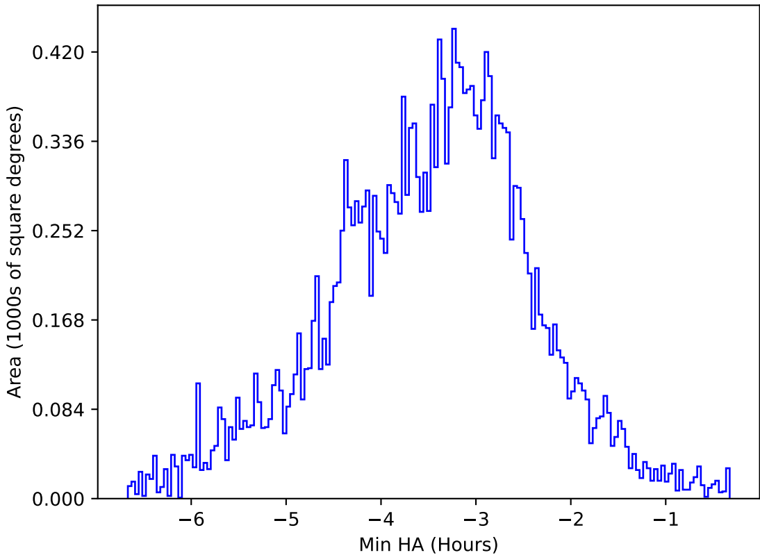
internal_u_expt27_nscale0.9v3.4_10yrs All sky y band: Min HA
