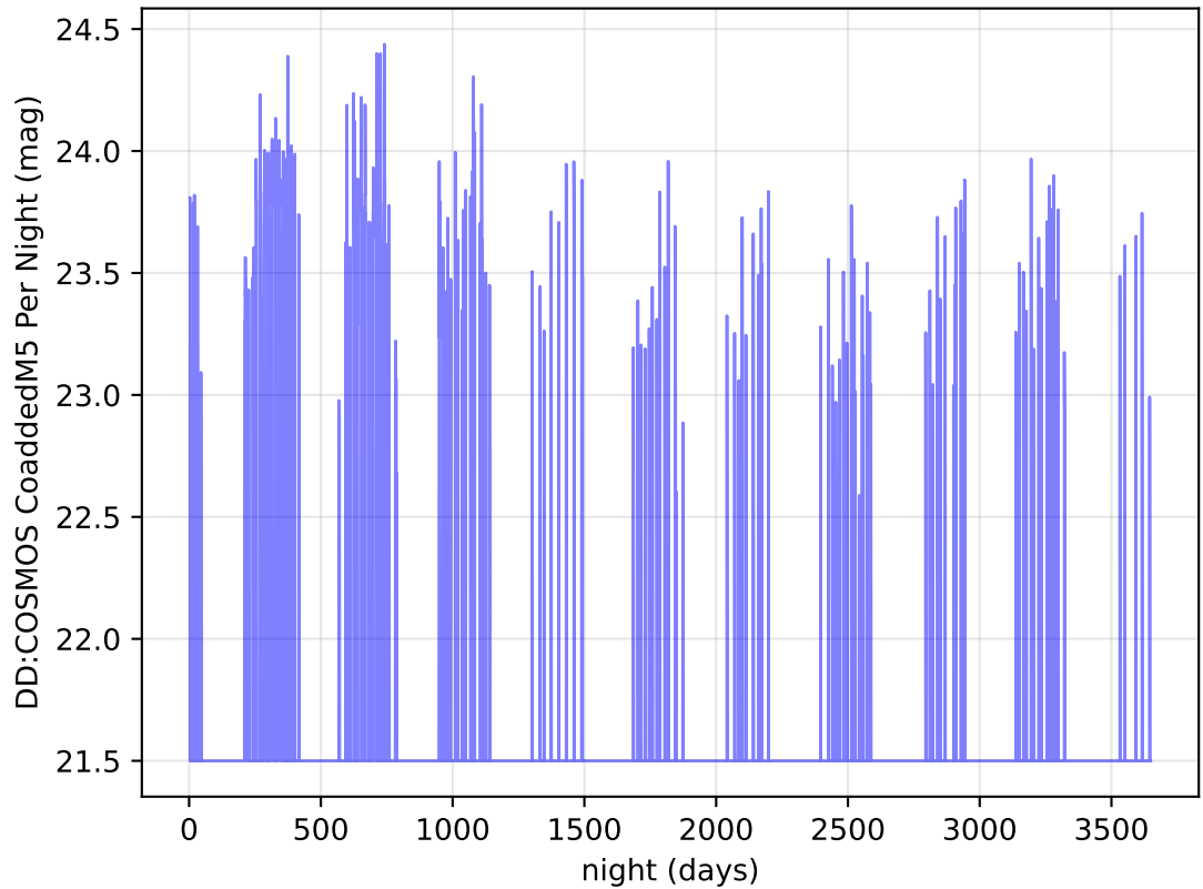
internal_u_expt27_nscale0.9v3.4_10yrs y band: DD:COSMOS CoaddedM5 Per Night
