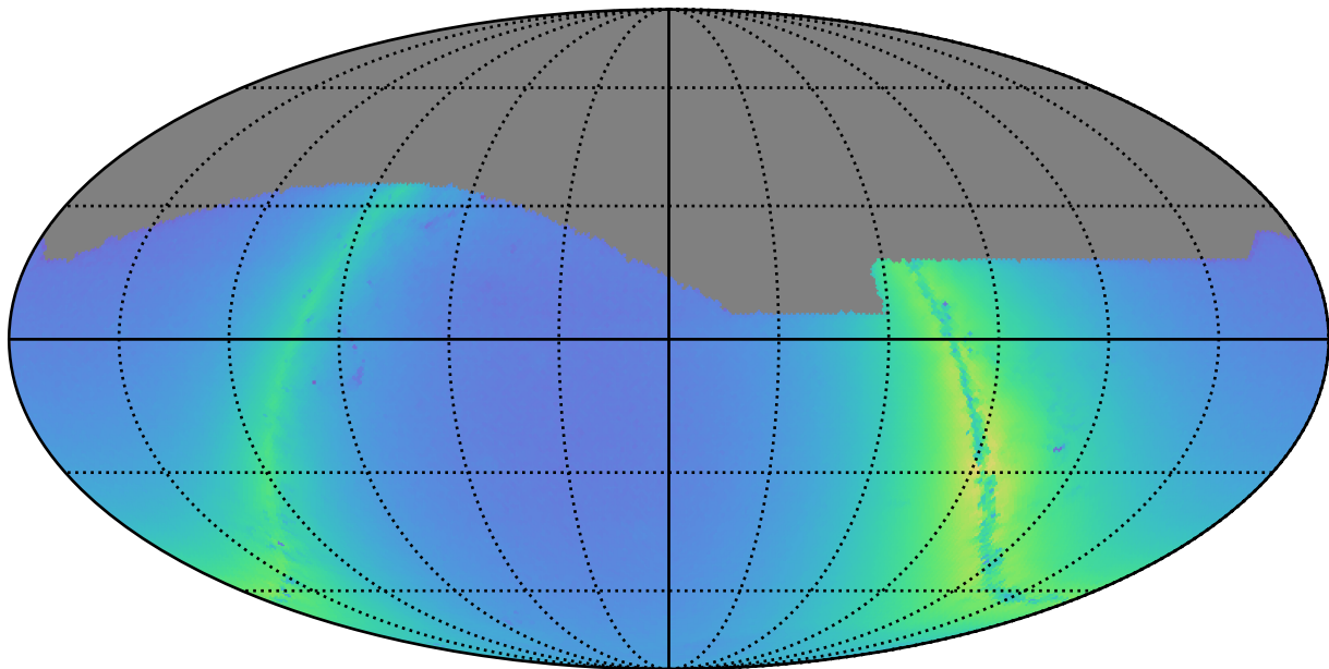
extra_ss_neo7_v3.4_10yrs r: Nstars_no_crowding
