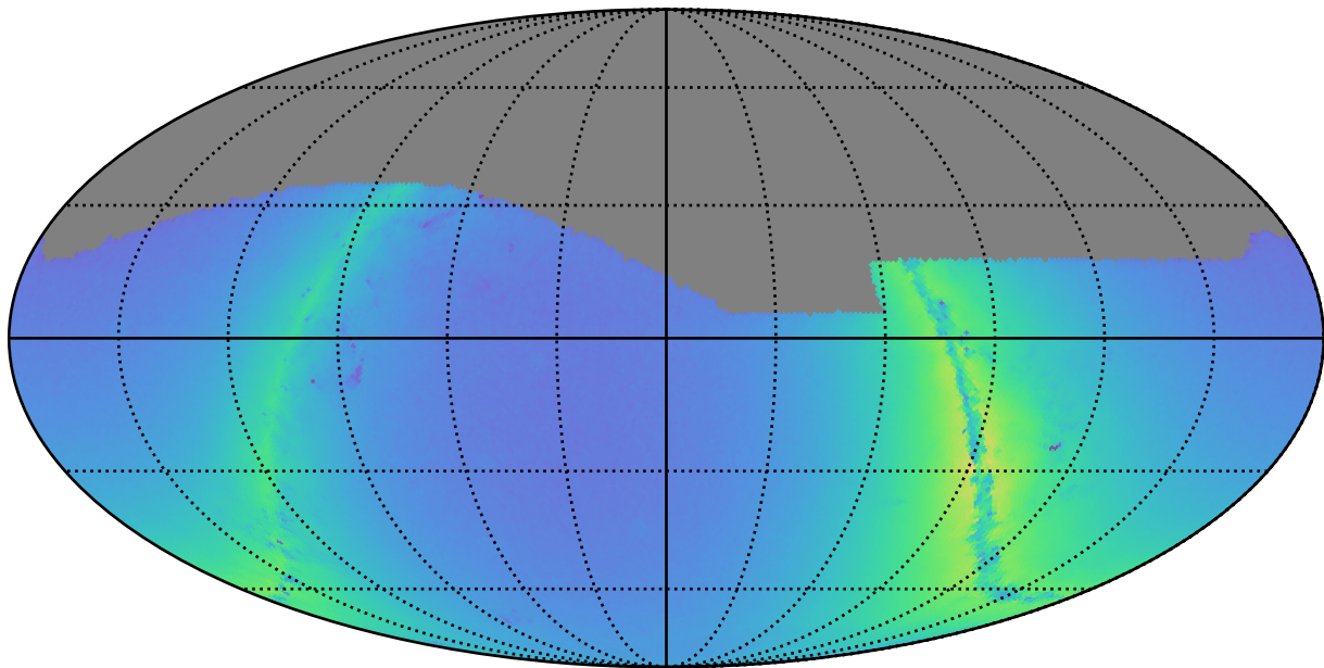
extra_ss_neo7_v3.4_10yrs g: Nstars_no_crowding
