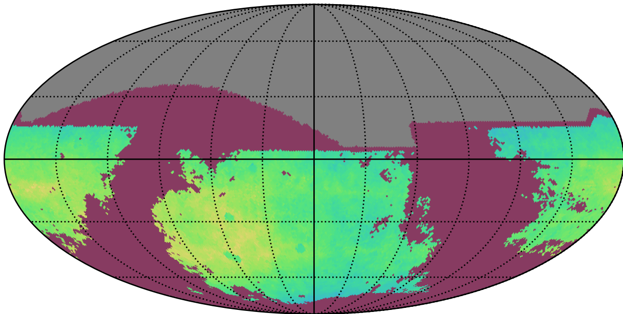
extra_ss_neo7_v3.4_10yrs i: NgalScale
