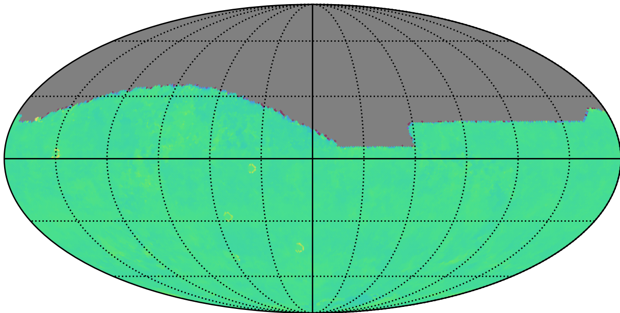
extra_ss_neo7_v3.4_10yrs z: Kuiper rotTelPos
