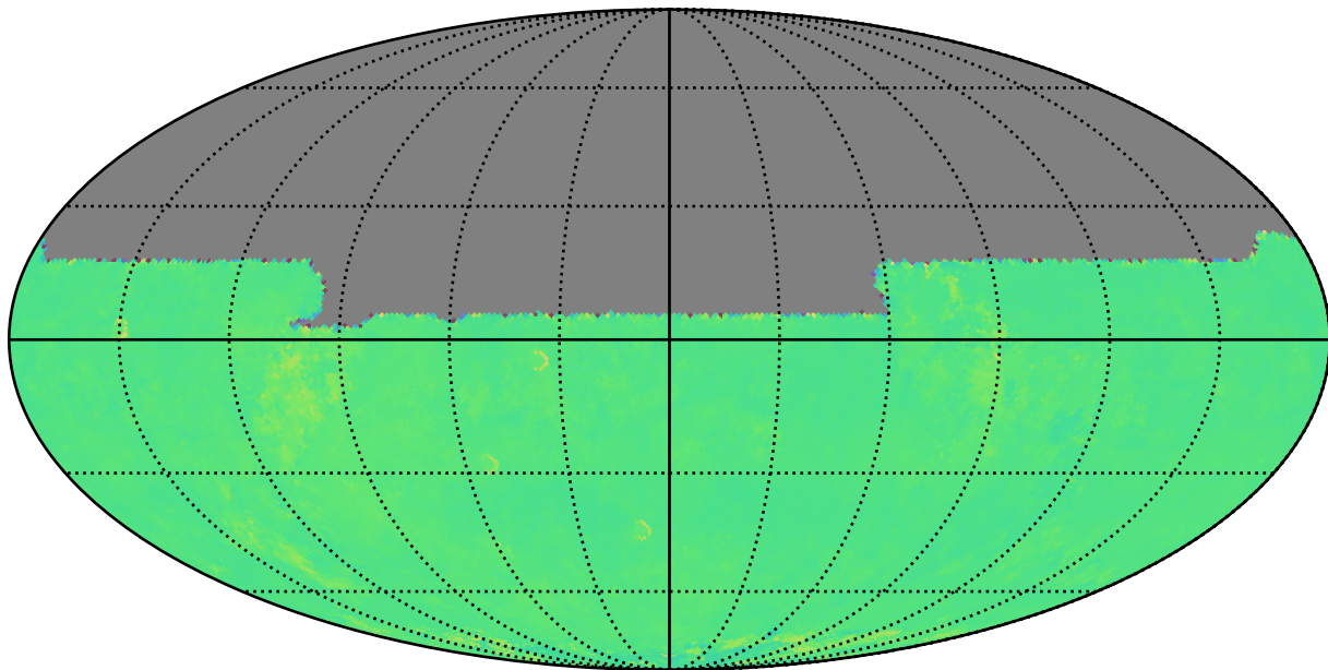
extra_ss_neo7_v3.4_10yrs y: Kuiper rotTelPos
