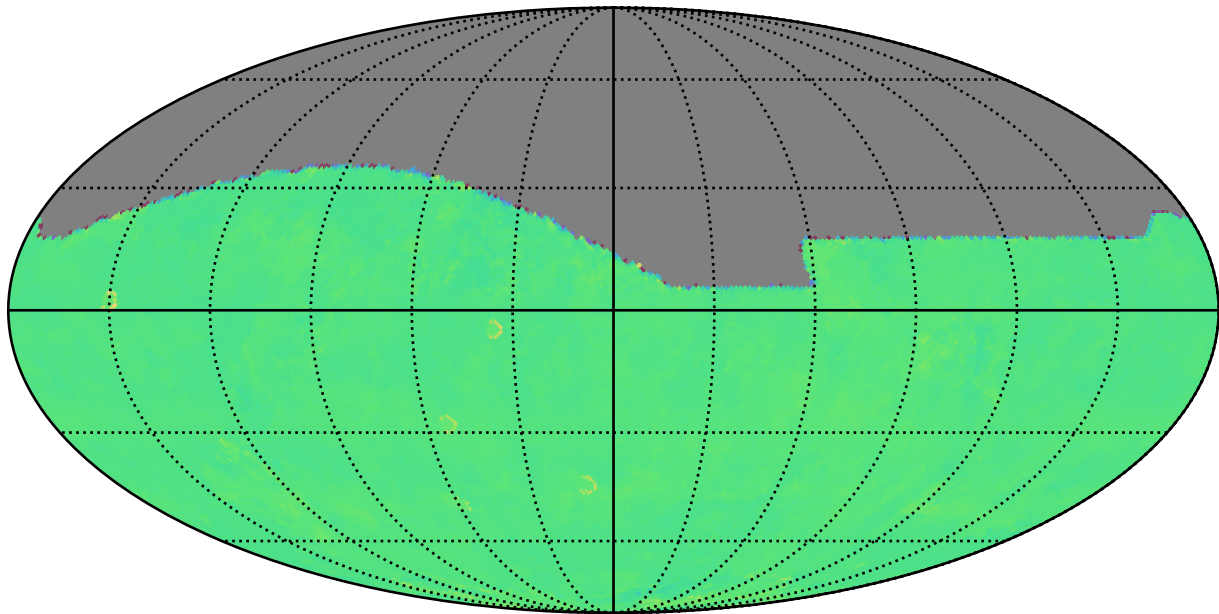
extra_ss_neo7_v3.4_10yrs r: Kuiper rotTelPos
