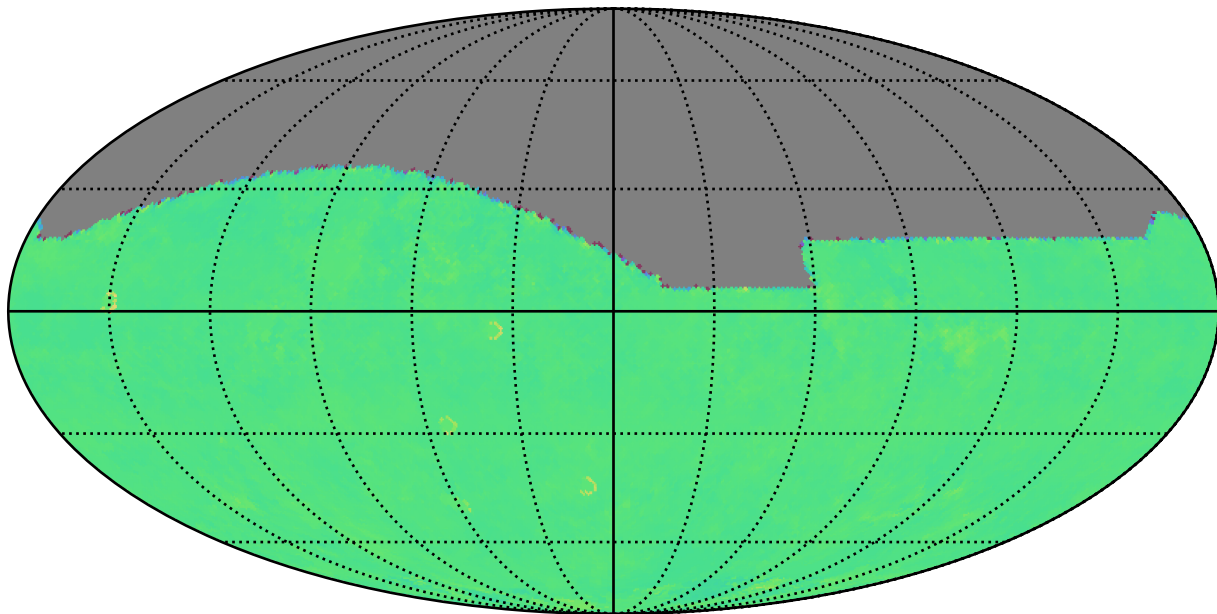
extra_ss_neo7_v3.4_10yrs i: Kuiper rotTelPos
